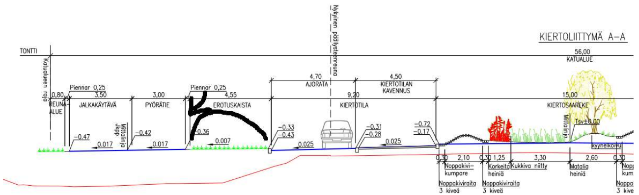
Kuva 3 Kuva 1 ojan tai painanteen (ja sen pohjalla olevan hulevesikaivon) sijaan viheralueen halutaan sulattavan lumet ja johtavan vedet jalkakäytävälle ja pyörätielle.
