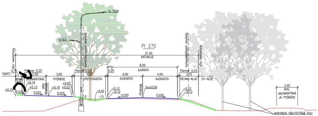
Kuva 2 Kuva 1 ojan tai painanteen (ja sen pohjalla olevan hulevesikaivon) sijaan viheralueen halutaan sulattavan lumet ja johtavan vedet jalkakäytävälle ja pyörätielle.
